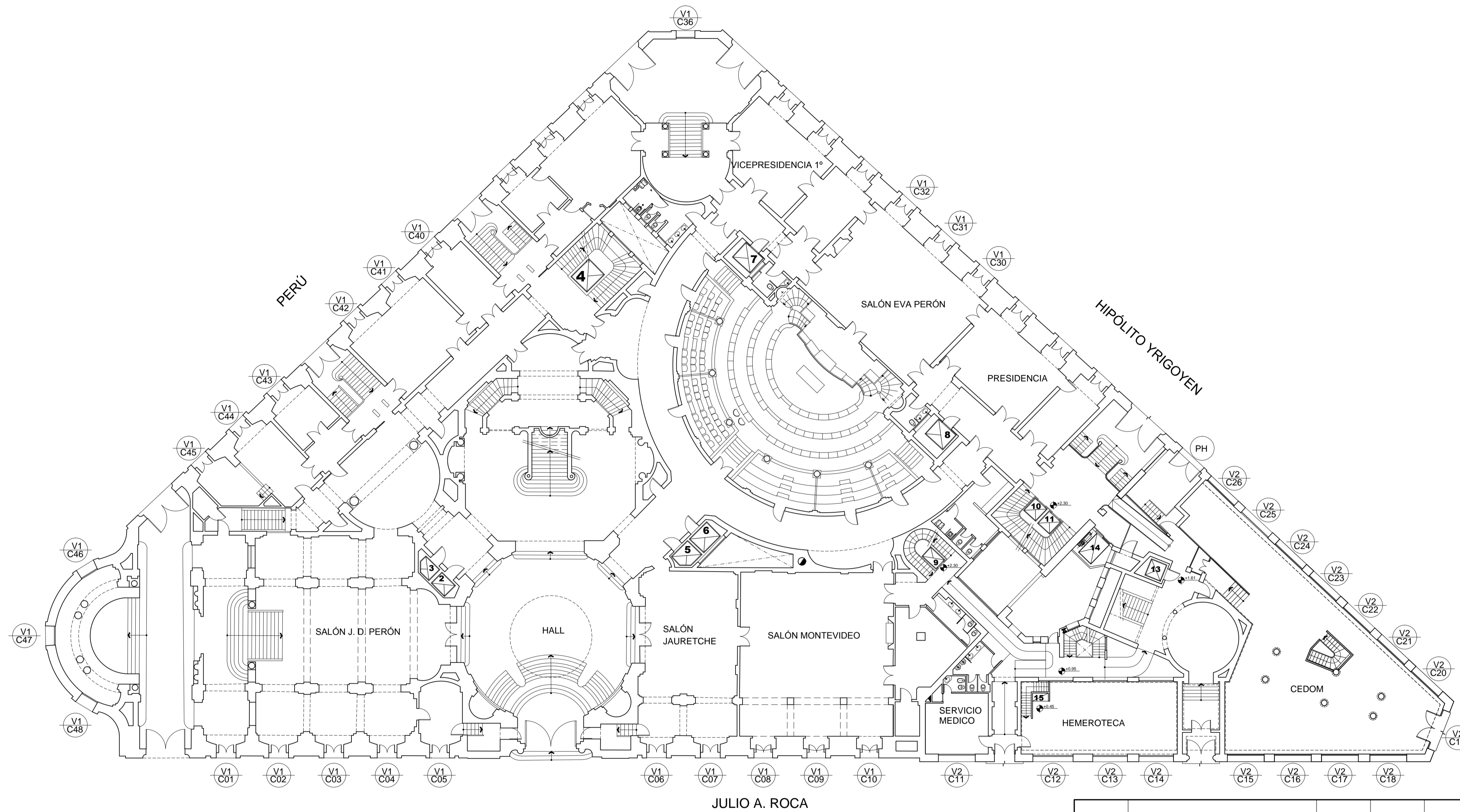
PLANTA BAJA 0 1 10 20
