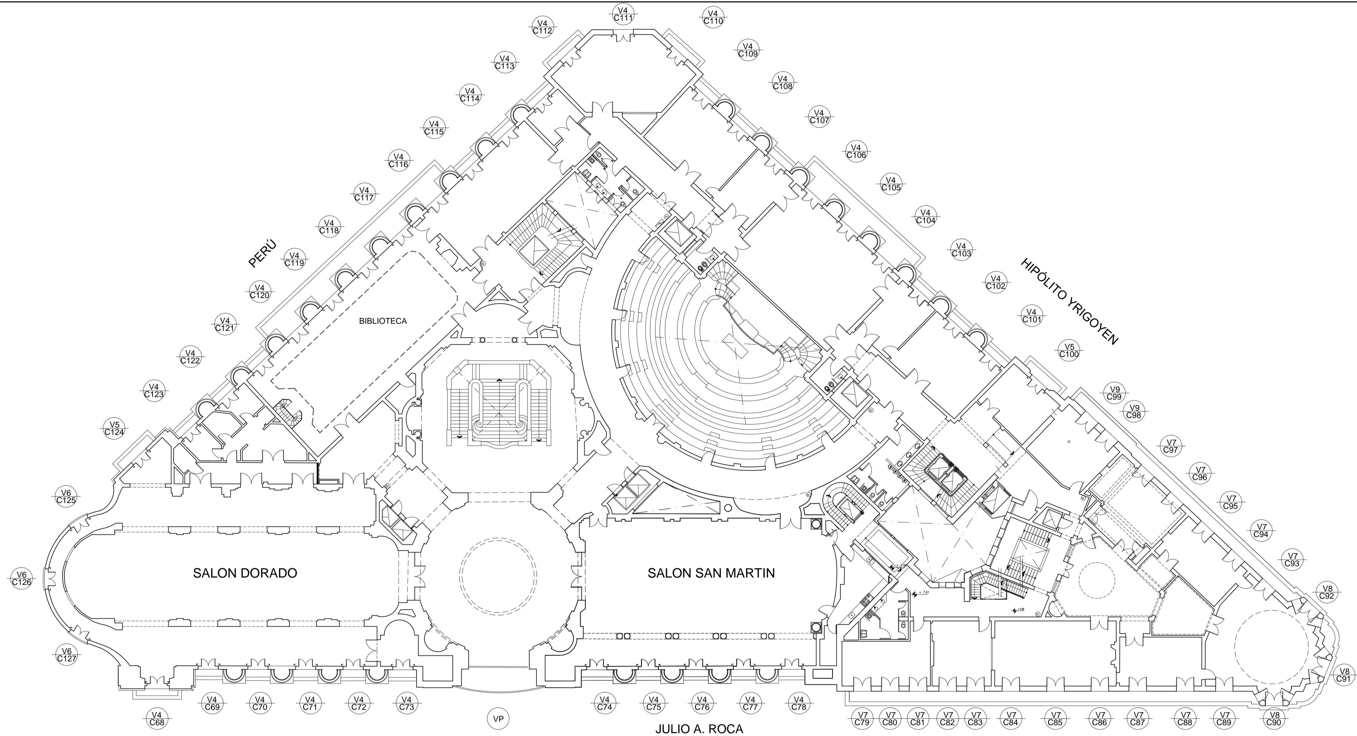
PLANTA PRINCIPAL 0 1 10 20
